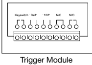
Trigger Module
